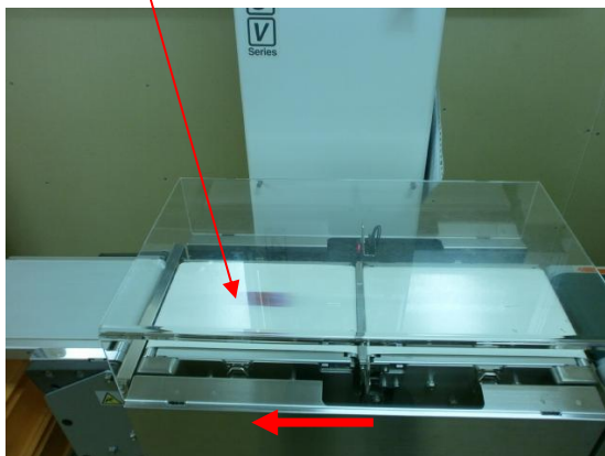
助走コンベアー(選別板への橋渡し)
